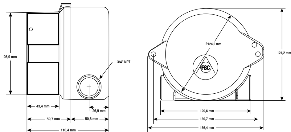
Allgemeine Abmessungen Seiten- und Rückansichten (alle Abmessungen in mm)
