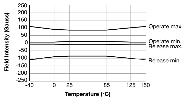
SS461/SS561AT
